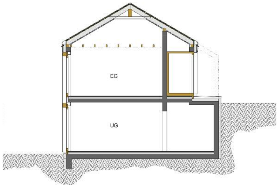
Schnitt durch das Schieferhaus am Hang
