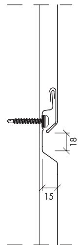
Paneelverbindung
